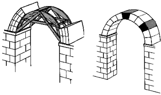
Romeinse boogconstructie
