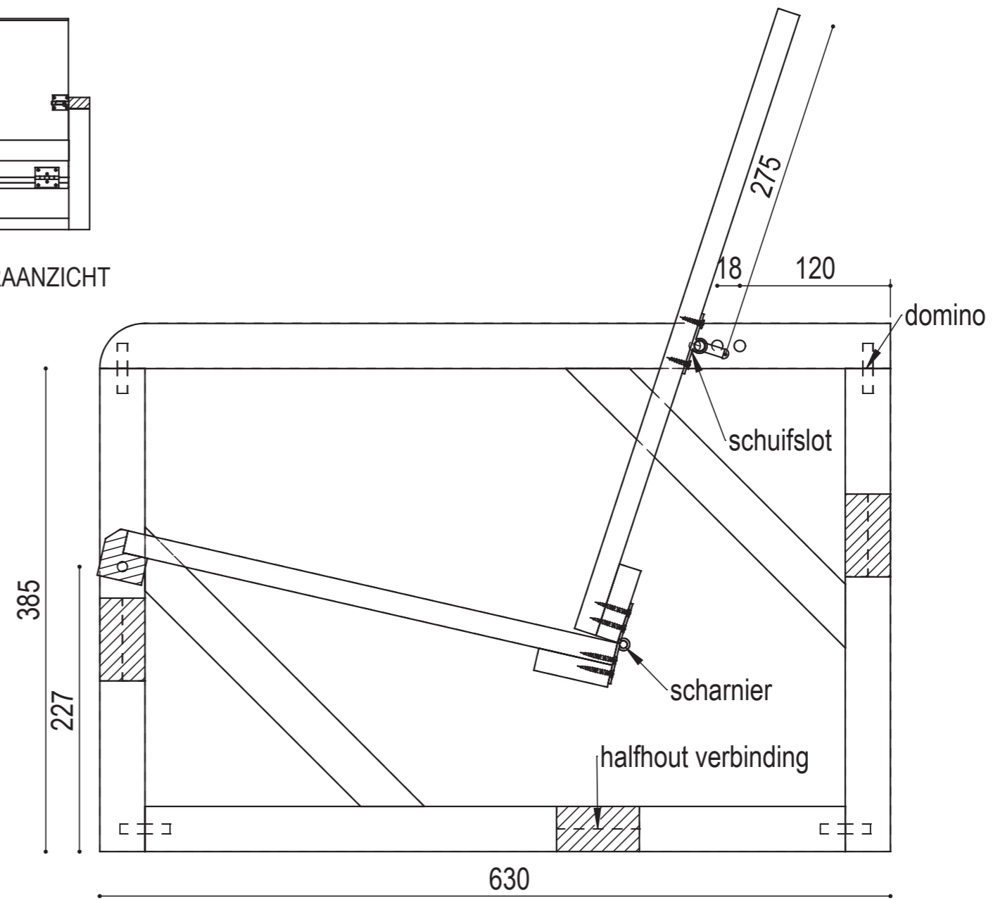
DOORSNEDE A-A
