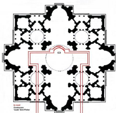
Afbeelding 08: Schets Plan van Bramante
