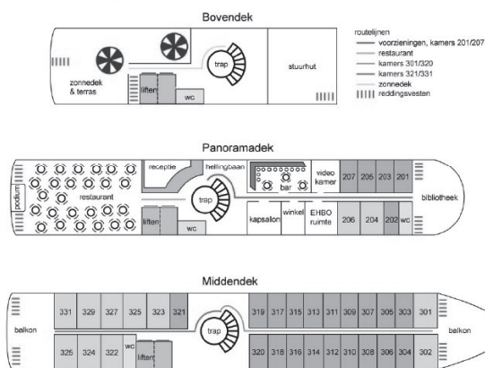
Bovenaanzicht De Pelikaan
