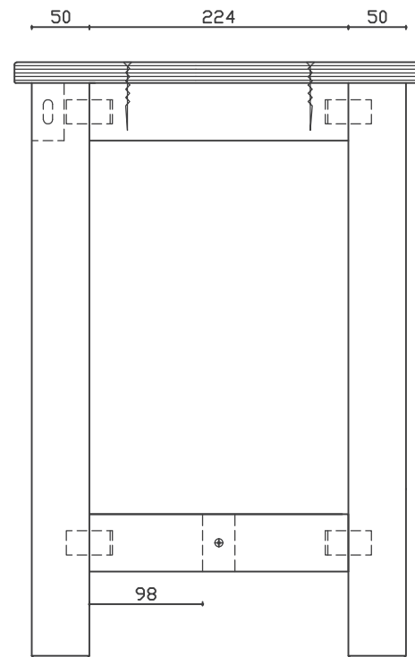
Zijaanzicht
