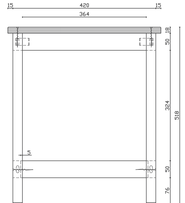
Vooraanzicht
