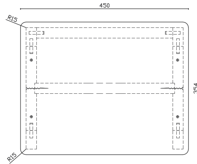
Bovenaanzicht
