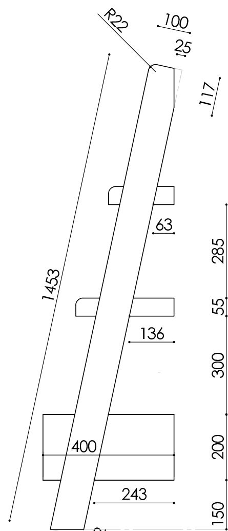
Rechterzijaanzicht
