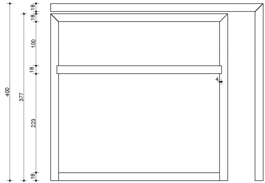
vooraanzicht
