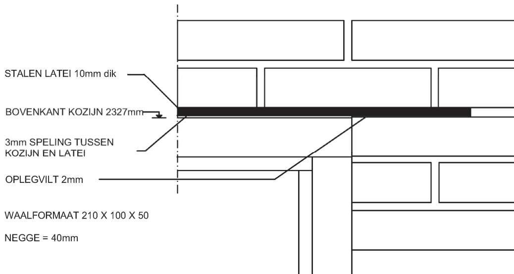
Detail bovenhoek kozijn en latei
